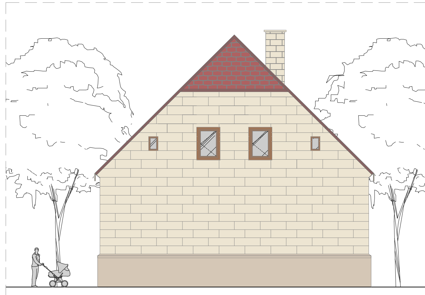
ELEWACJA BOCZNA
