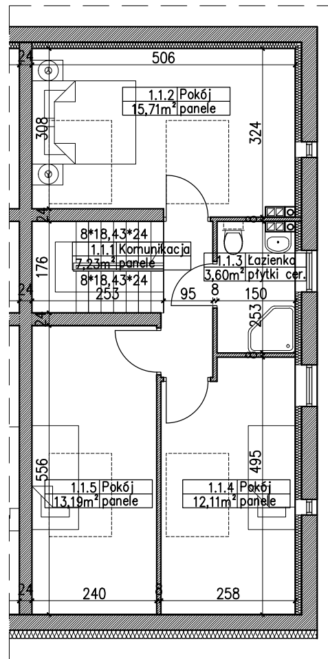
PIĘTRO - 51,84m 2
